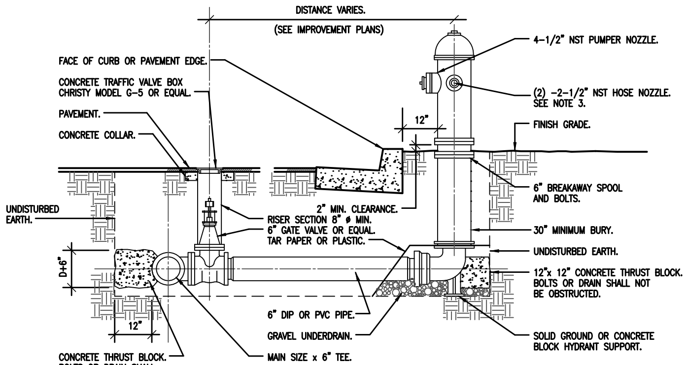
ELEVATION
